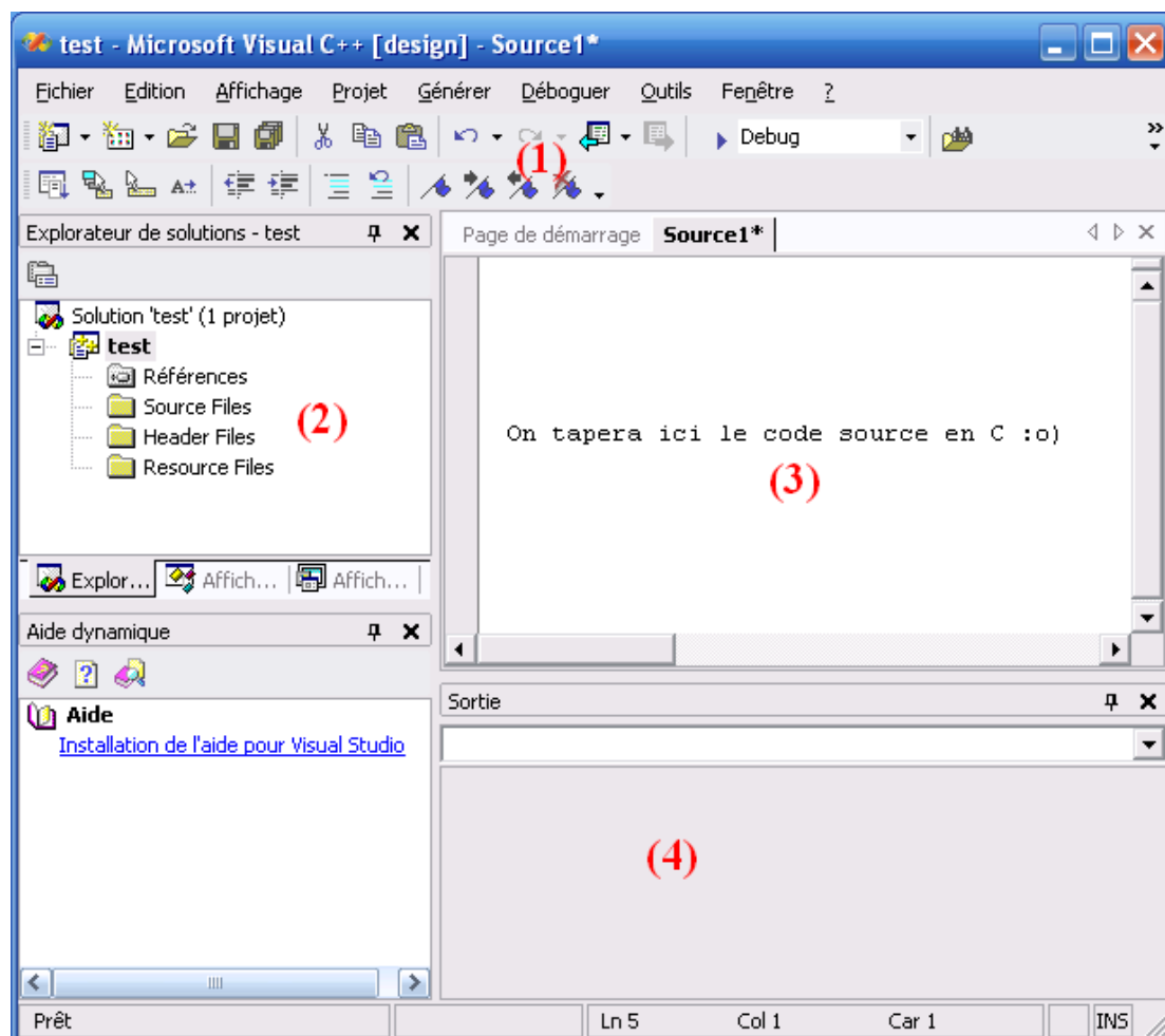
Visual C++ en détail
